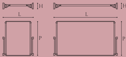
TELAIO ESTRAIBILE INTERNO PER MODULO 1/A E 2/A PULLOUT FRAME FOR 1-2 DOORS UNIT / ТЕЛЕСКОПИЧЕСКАЯ РАМА ПОЛНОГО ВЫДВИЖЕНИЯ ДЛЯ 1-2-СТВ. МОДУЛЕЙ
