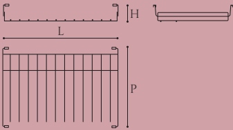
PORTAPANTALONI INTERNO PER MODULO 2/A PULLOUT TROUSERS RACK FOR 2 DOORS UNIT / ВЫДВИЖНАЯ ВЕШАЛКА ДЛЯ БРЮК ДЛЯ 2-СТВ. МОДУЛЯ
