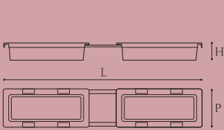
VASCHETTA MULTIUSO INTERNA PER MODULO 2/A MULTI-PURPOSE TRAY FOR 2 DOORS UNIT / УНИВЕРСАЛЬНЫЙ ЛОТОК ДЛЯ 2-СТВ. МОДУЛЕЙ
