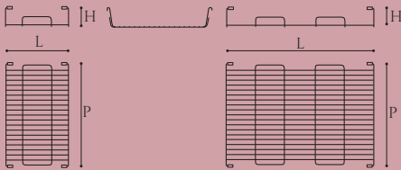
CESTO INTERNO PER MODULO 1/A E 2/A PULLOUT BASKET FOR 1-2 DOORS UNIT / ВЫДВИЖНАЯ КОРЗИНА ДЛЯ 1-2-СТВ. МОДУЛЕЙ
