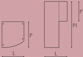
PER COLONNA TERMINALE (A) O PER MODULO CABINA ANGOLO (B) FOR END COLUMN (A) OR CORNER UNIT (B) / ДЛЯ ЗАВЕРШАЮЩЕГО МОДУЛЯ (A) ИЛИ ДЛЯ УГЛОВОВО ШКАФА (B)
